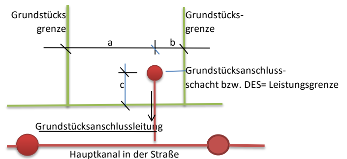
Prinzipskizze
