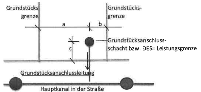
Prinzipskizze
