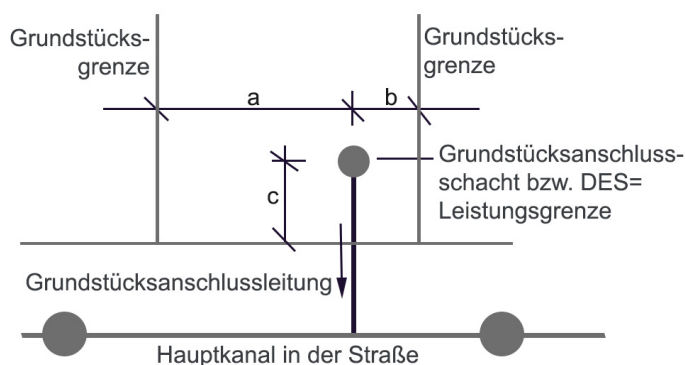
Prinzipskizze
